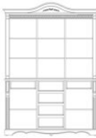
Тумба «Паола 2105» БМ670: L1550xВ463xH903 Секция-витрина 3д «Паола 2106» БМ670: L1612xВ468xH1226
