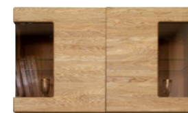
Шкаф навесной «Хедмарк 2248Бр» БМ760: L1201xB442xH700
