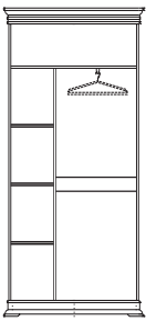
Шкаф «Верди Люкс 2/2» П487.35: L1148xB477xH1996 (с выдвижной штангой для плечиков)
