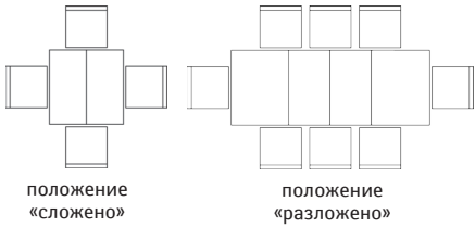
Стол «Тунис 14» П352.03: L900/2400xB900xH779
