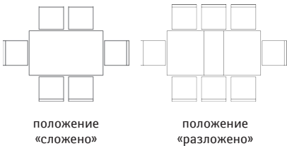
Стол обеденный «Юстина 2337» БМ694: L1640xВ870xH766 В разложенном виде 2134x870
