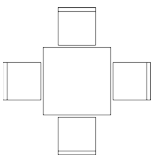
Стол «Тунис 1» П352.01: L900xB900xH777
