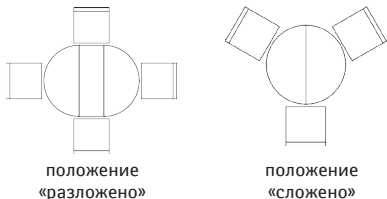
Стол «Верди 12А» П318.07: L1100/1450xВ1100xH778
