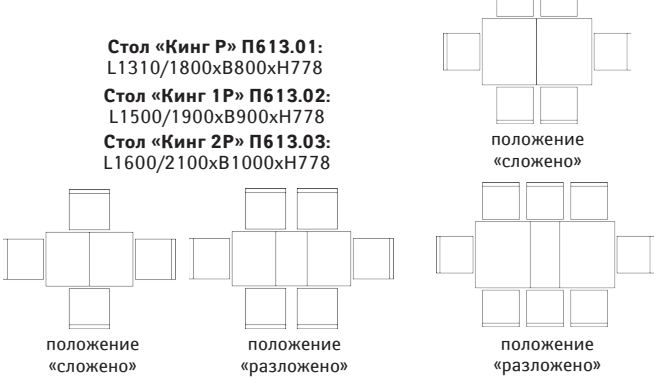
Стол «Кинг 14» П613.07: L1600/2100/2600/3100xВ1000xH778
