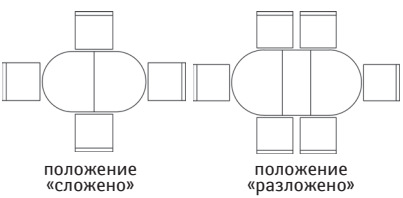
Стол «10А» П313.14: L1410/1900xВ900xH778
