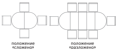
Стол «14А» П323.12: L1300/1770/2240/2710xВ1000xH778 Стол «14/1А» П323.14: L1030/1460/1890/2320xВ1030xH778
