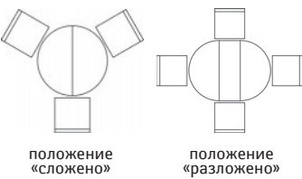
Стол «12А» П318.14: L1100/1450xВ1100xH778
