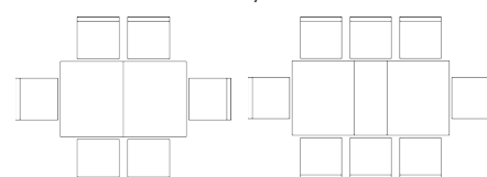
Стол «Альба 1Р» П498.02: L1500/1900xВ900xH778
