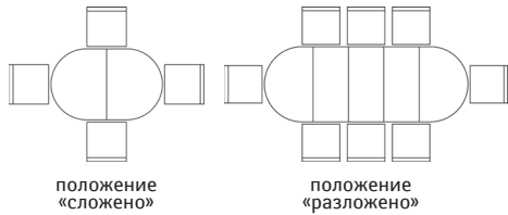
Стол «14» П323.11: L1300/1770/2240/2710xВ1000xH778
