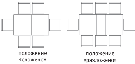
Стол «Тунис 1Р» П352.02: L1500/1900xB900xH777
