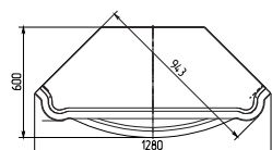
Размер проёма L410xH605 встраиваемая глубина камина - 144 мм
