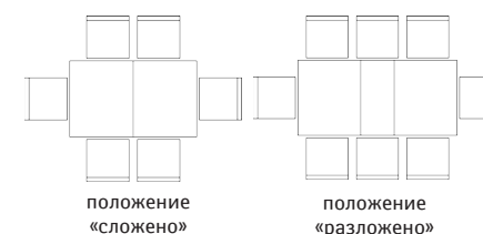
Стол «Алези 3Р» П353.08: L1500/1900xВ900xH757
