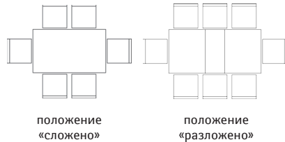
Стол обеденный «Паола 2158» БМ674: L1640 x B870 x H766 В разложенном виде 2140 x 870 x 766
