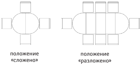
Стол «Милана 14» П323.02: L1300/1770/2240/2710xВ1000xH778
