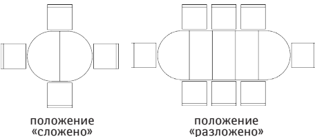
Стол «Верди 14/1А» П323.09: L1030/1460/1890/2320xВ1030xH778
