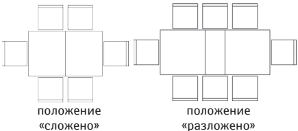
Стол «Верди 1Р» П106.04: L1800/2200xВ900xH775
