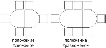
Стол «Валенсия 18» П394.03: L1800/2300xВ1100xH762
