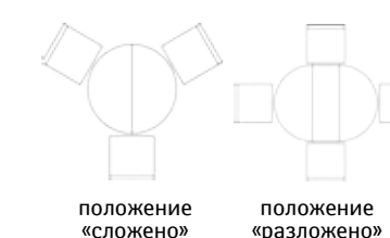
Стол «Милана 12А» ПЗ18.08: L1100/1450xВ1100xH778
