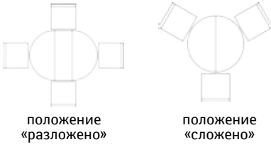
Стол «Верди 12А» П318.07: L1100/1450xB1100xH778
