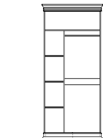
Шкаф «Верди Люкс 2/3» П487.36: L1148xB637xH1996
