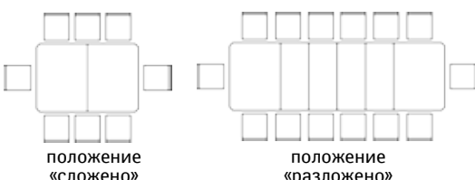
Стол «Верди 28» П394.04: L1800/3800xB1200xH777
