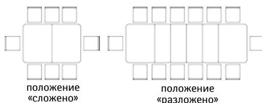
Стол «Верди 38» П394.10: L2000/4000xB1200xH777
