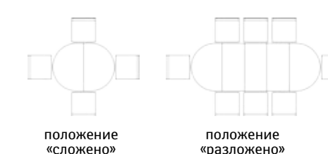
Стол «Милана 14» ПЗ23.02: L1300/1770/2240/2710xВ1000xH778
