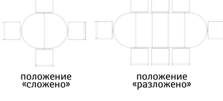
Стол «14А» П323.12: L1300/1770/2240/2710xB1000xH778
