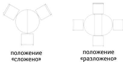
Стол «Верди 11/1» П317.04: L800/1100xB800xH778
