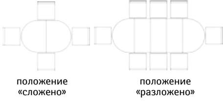
Стол «Верди 14» П323.01: L1300/1770/2240/2710xB1000xH778
