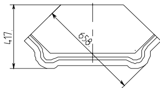
Полка «Алези 1 Люкс» П350.21Л: L1540xВ220xH1222
