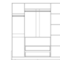
ШКАФ ДЛЯ ОДЕЖДЫ П631.01: L2023xВ581xH2200
