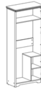
Шкаф для одежды П047.1103: L850xВ430xH2050
