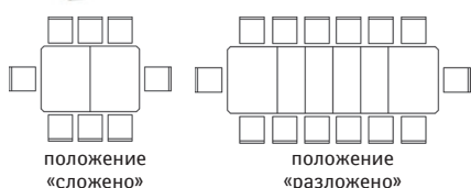
Стол «Верди 28» P394.04: L1800/3800xB1200xH777
