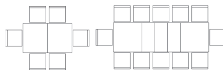
Стол «Алези 14Р» П353.09: L1700/3200xВ1100xH757
