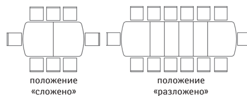
Стол «Валенсия 38» П394.12: L2000/4000xВ1200xH777
