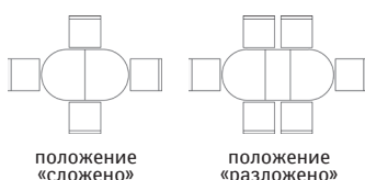
Стол «Верди 5РД» P106.16: L1380/1780xB800xH740
