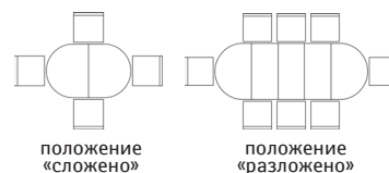
Стол «Верди 14» П323.01: L1300/1770/2240/2710xВ1000xH778
