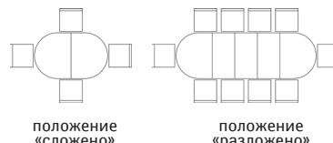
Стол «Верди 4РД» P106.15: L1600/2100/2600/3100xB1000xH770
