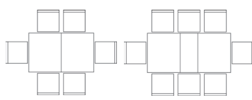
Стол «Алези 2РЕ» П353.06: L1500/1900xВ900xH777
