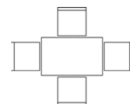
Стол обеденный «Моника» П4.646.4.07: L1100xB700xH776 Стол обеденный «Моника» П4.646.4.00: L1200xB800xH776
