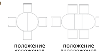
Стол обеденный «Лагус» БМ2.805.4.42: L1290xВ1290xН760 В разложенном виде: L1680xВ1290xН760
