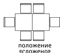
Стол обеденный «Моника» (с механизмом) П4.646.4.02-Р: L1600/2000xВ900xH777 Стол обеденный «Моника» (с механизмом) П4.646.4.03-Р: L1800/2200xВ1000xH777
