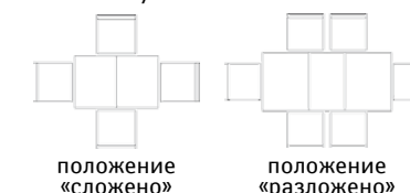
Стол обеденный «Поло» П4.257.4.07: L1310/1800xВ800xH766
