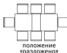
Стол обеденный «Моника» (с механизмом) П4.646.4.02-Р: L1600/2000xВ900xH777 Стол обеденный «Моника» (с механизмом) П4.646.4.03-Р: L1800/2200xВ1000xH777
