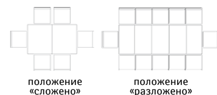
Стол обеденный «Кинг» П4.193.4.07: L1600/2100/2600/3100xВ1000xH778
