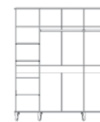
Шкаф для одежды 4д «Флорентина» БМ2.851.1.27-01: L1936xВ630xH2178
