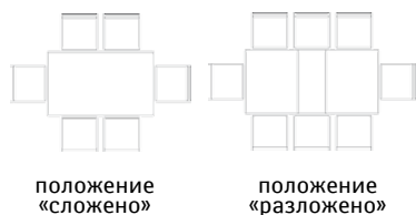
Стол обеденный «Юстина» БМ2.691.4.42: L1640xB870xH766 в разложенном виде: L2134xB870xH766
