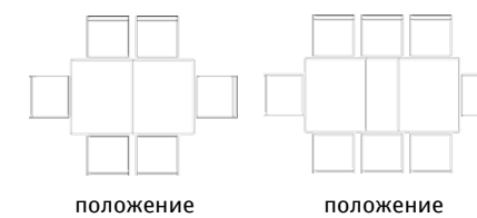
Стол обеденный «Алыт» П6.490.4.22: L1500/1900xВ900xH776 Стол обеденный «Алыт» П6.490.4.23: L1100/1490xВ900xH776
