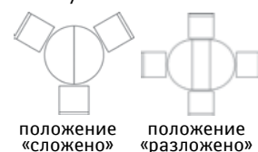
Стол обеденный «Валенсия Классик» ПЗ.0589.4.12: L1100/1450xВ1100xH778
