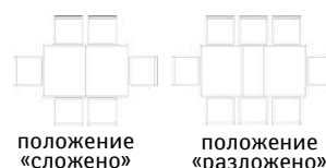
Стол обеденный «Версаль» БМ2.777.4.42: L1640/2134xB870xH759
