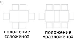
Стол журнальный «Кармен Прованс» ПЗ.0581.0.03: L1200xВ700xH450
