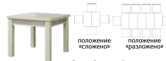
Стол обеденный «Тунис» П6.343.4.03: L900/2400xB900xH777
