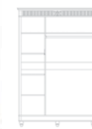
Шкаф для одежды 3д «Юстина» БМ2.691.1.03-01: L1500xB636xH2250
